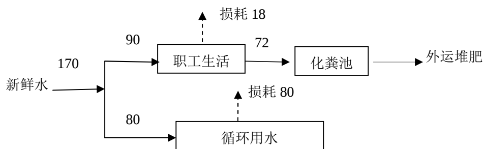
图 3-1 本项目水平衡图 (t/a)
