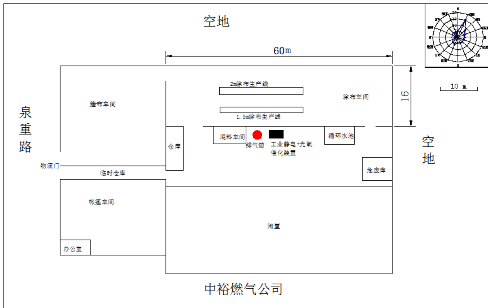
附图 4 项目平面布置示意图
