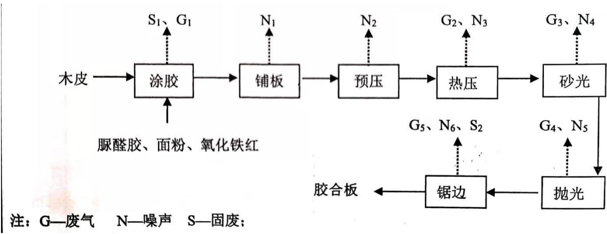
图 3.5-1 胶合板生产工艺流程及产污环节图
