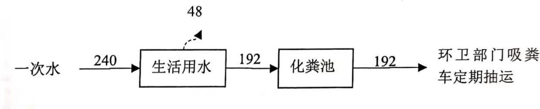
图 3.4-1 水量平衡图（m³/a）
