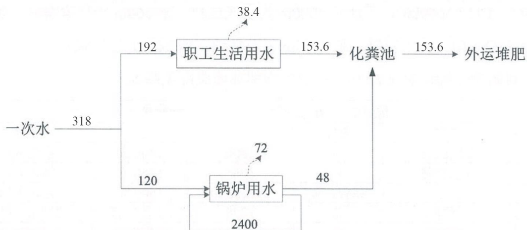
图 3-1 本项目水平衡图 单位： \text{m}^3/\text{a}
