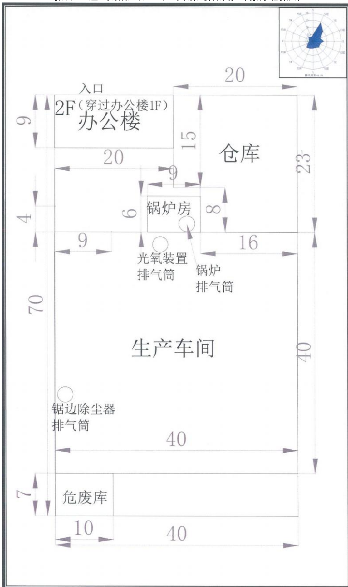
附图 3.本项目平面布置图
