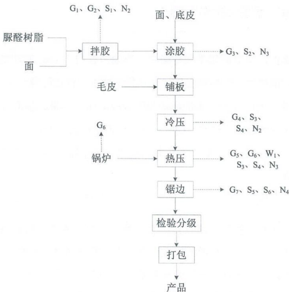
图 3-2 项目生产工艺流程及产污环节图
