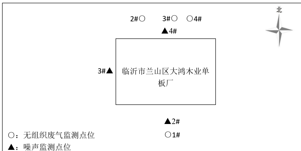
图 7-1 厂界噪声、无组织废气检测布点示意图 (2021-09-15)
