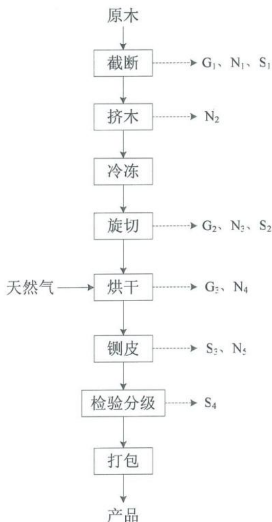
图 3-2 项目生产工艺流程及产污环节图
