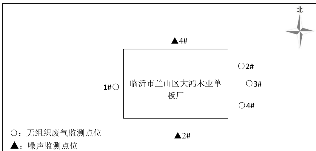
图 7-2 厂界噪声、无组织废气检测布点示意图（2021-09-16）
