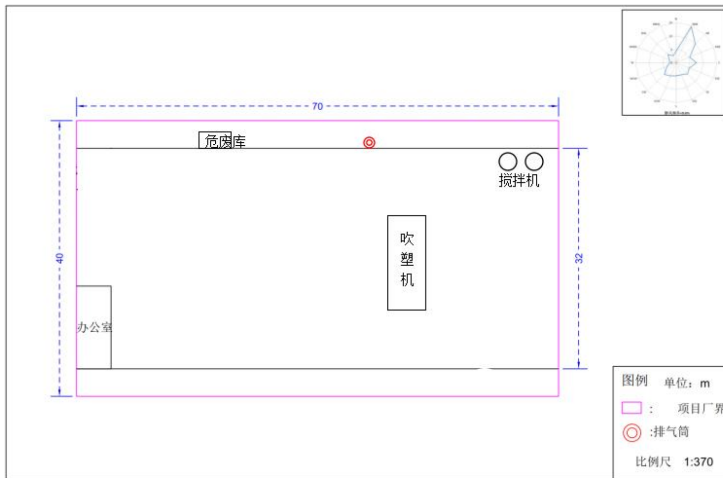
图 3-4 厂区平面布置图
