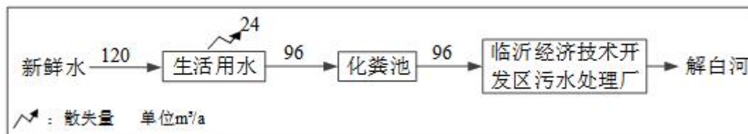
图 3-5 本项目水平衡图 ( \text{m}^3/\text{a} )
