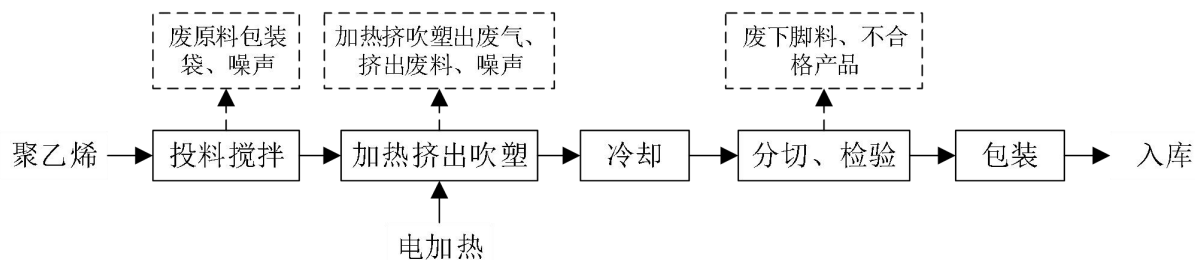
图 3-6 本项目塑料包装膜工艺流程及产污环节图
