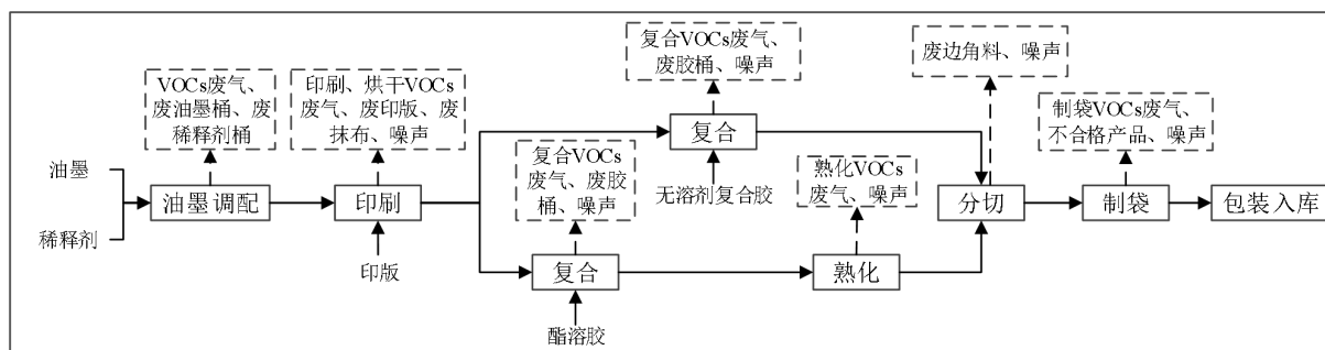
图 3-6 本项目各类包装袋工艺流程及产污环节图
