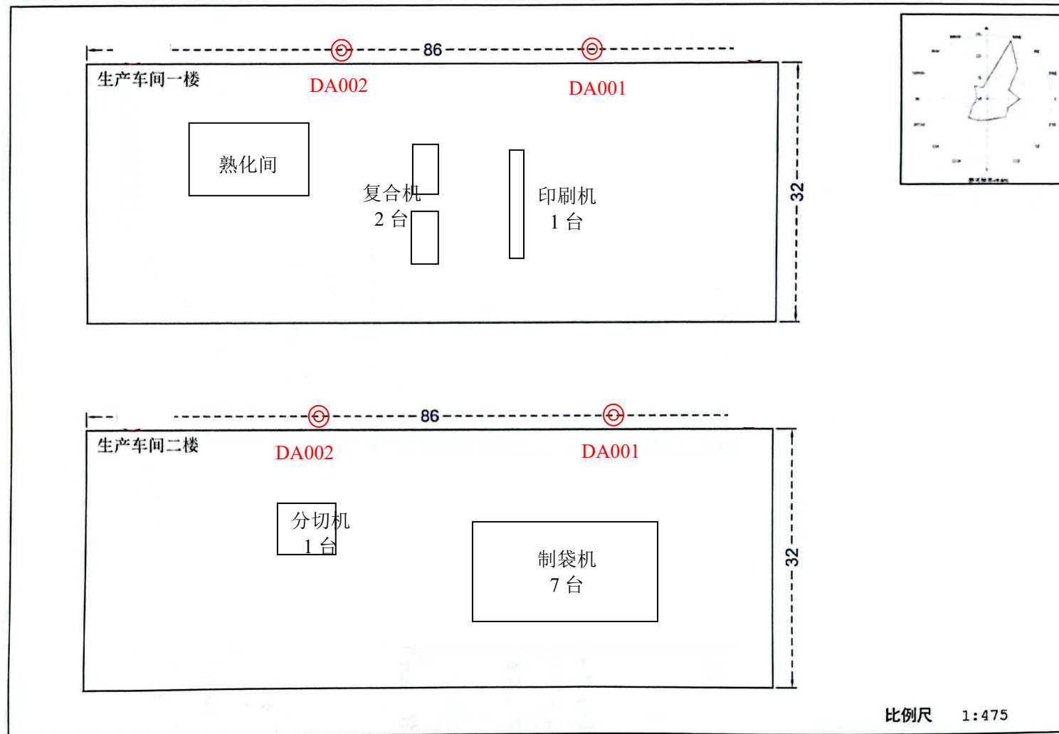
图 3-4.2 生产车间平面布置图
