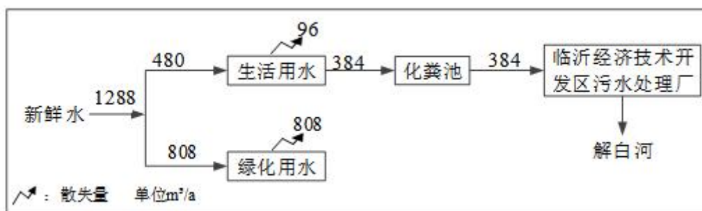
图 3-5 本项目水平衡图 (m 3 /a)
