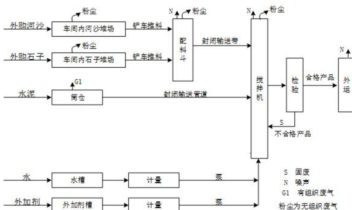
图 3.5-1 混凝土生产工艺流程及产污环节图
