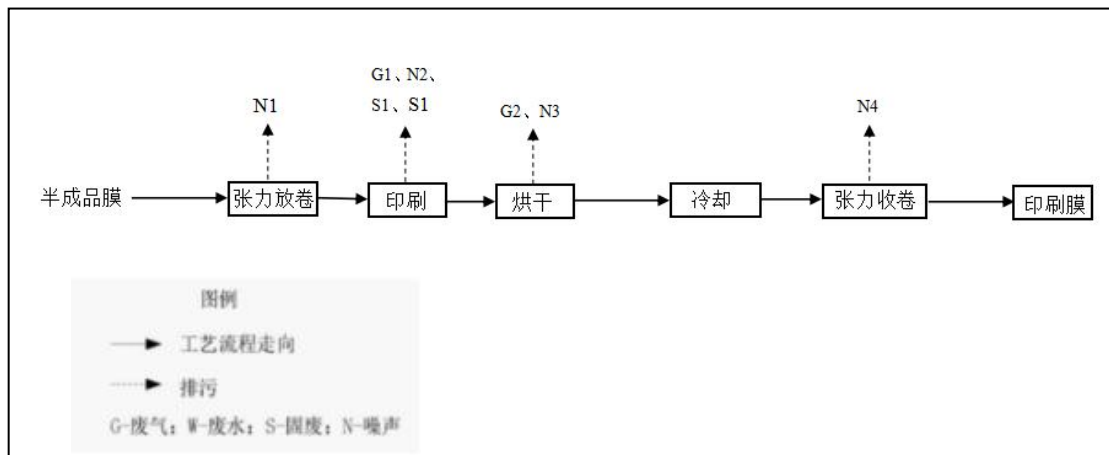
图 3-6 项目三期工艺流程及产污环节图
